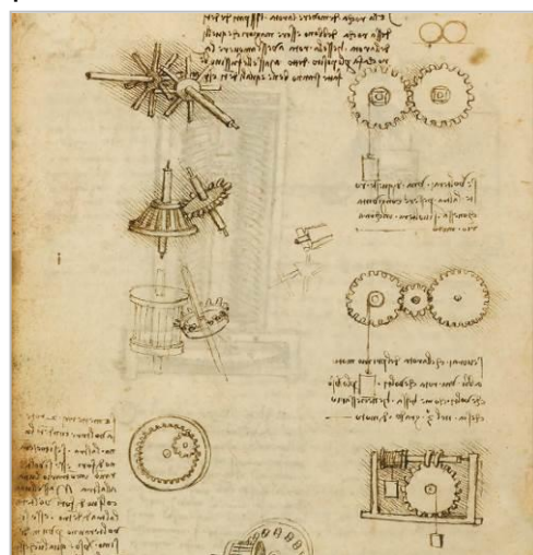
Foli f 15v. Còdex Madrid I (Ms. 8937). «Tractat d'estàtica i mecànica». 192 folis (384 pàg.) Format interior: 215 x 145 mm Mecànica aplicada (màquines i enginys) Mecànica aplicada (components) Principis de mecànica, cinemàtica, dinàmica Crèdit: Album
