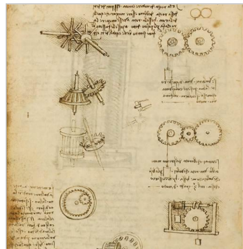
Foli f 15v. Còdex Madrid I (Ms. 8937). «Tractat d'estàtica i mecànica». 192 folis (384 pàg.) Format interior: 215 x 145 mm Mecànica aplicada (màquines i enginys) Mecànica aplicada (components) Principis de mecànica, cinemàtica, dinàmica Crèdit: Album
